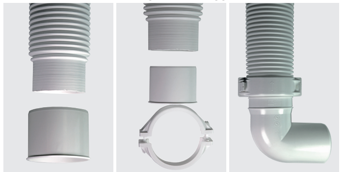
Illustrazione dei dettagli di montaggio raccordo PFA
