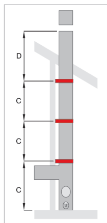
Sistema camino a vista appoggiato su di un basamento
